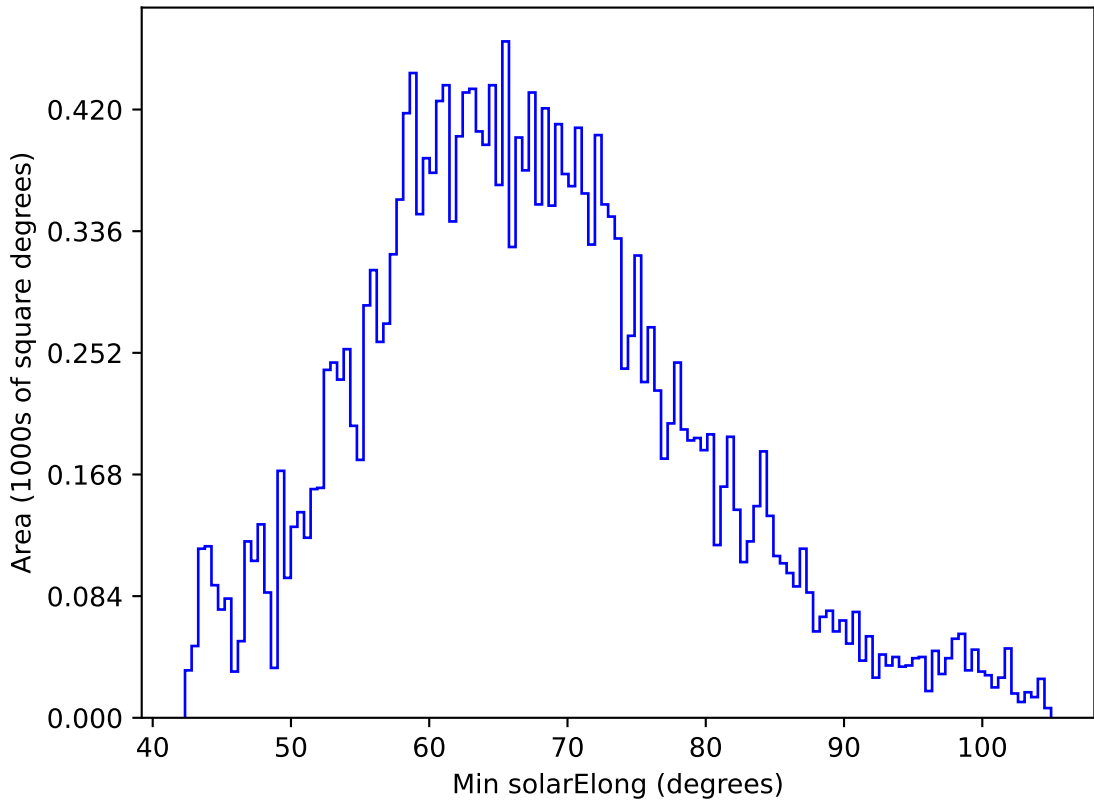
ddf_acor_sf10_lsf20_lsr50_v3.4_10yrs All sky y band: Min solarElong
