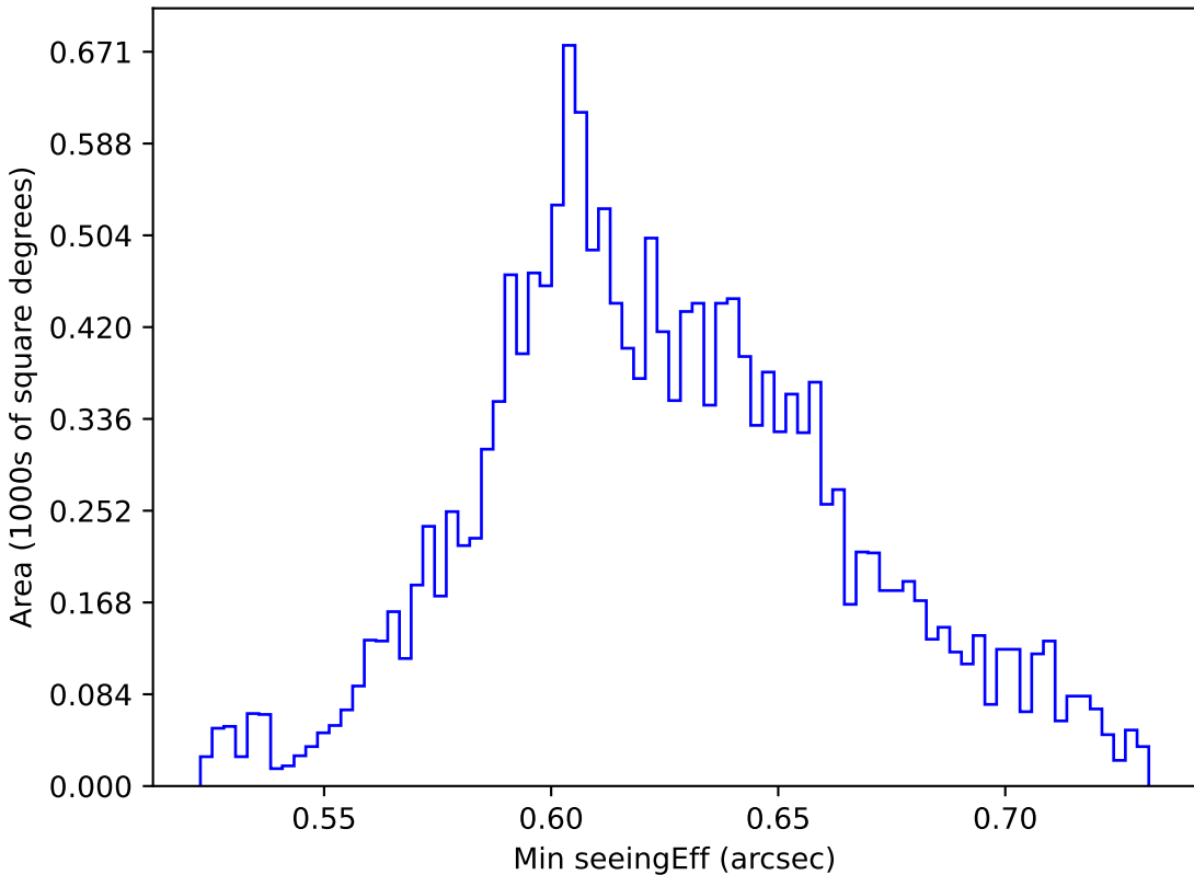
ddf_acor_sf10_lsf20_lsr50_v3.4_10yrs WFD y band: Min seeingEff
