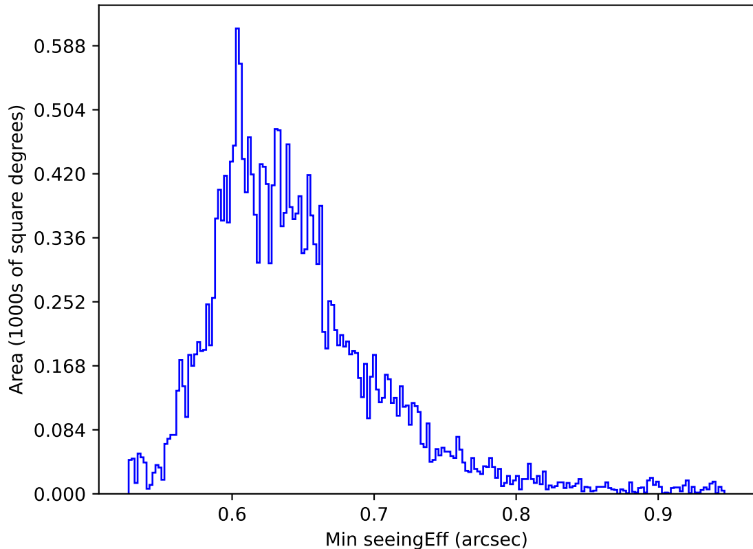
ddf_acor_sf10_lsf20_lsr50_v3.4_10yrs All sky y band: Min seeingEff
