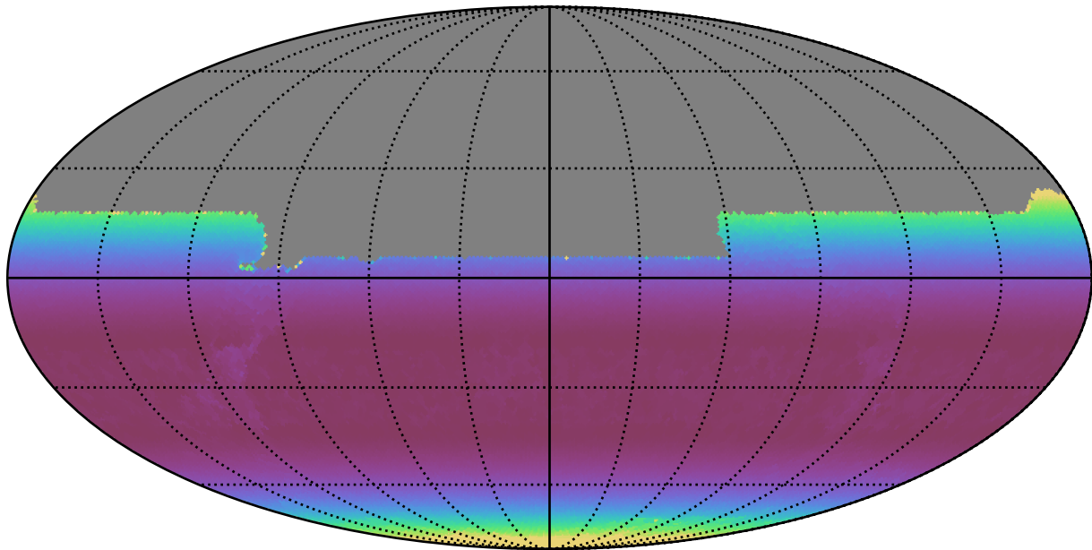
ddf_acor_sf10_lsf20_lsr50_v3.4_10yrs All sky y band: Min airmass
