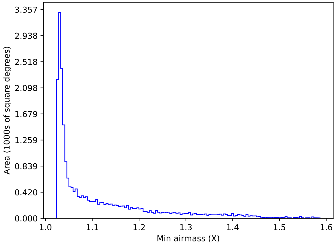
ddf_acor_sf10_lsf20_lsr50_v3.4_10yrs All sky y band: Min airmass
