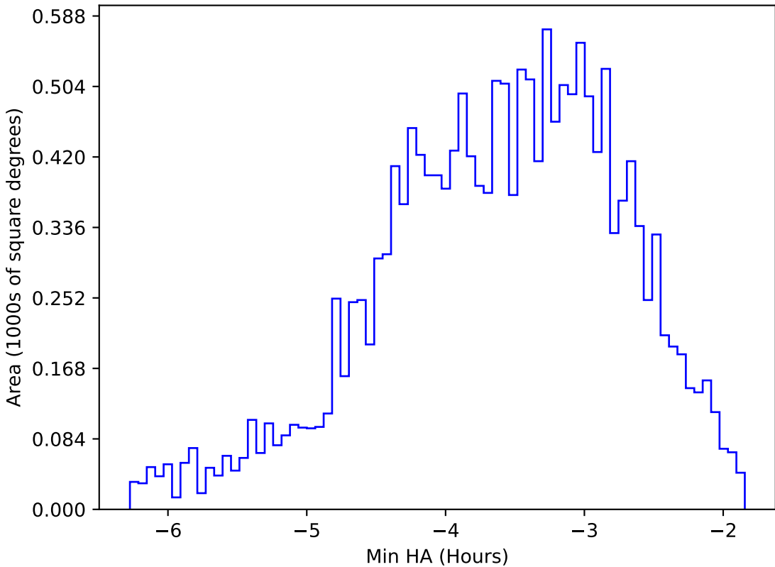
ddf_acor_sf10_lsf20_lsr50_v3.4_10yrs WFD y band: Min HA
