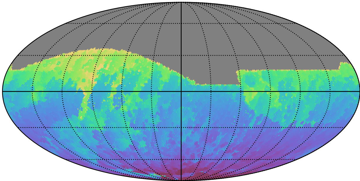
ddf_acor_sf10_lsf20_lsr50_v3.4_10yrs All sky z band: Min HA
