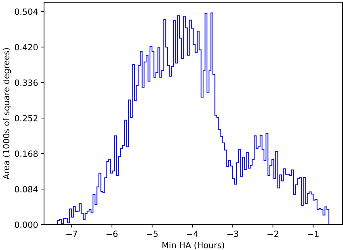
ddf_acor_sf10_lsf20_lsr50_v3.4_10yrs All sky z band: Min HA
