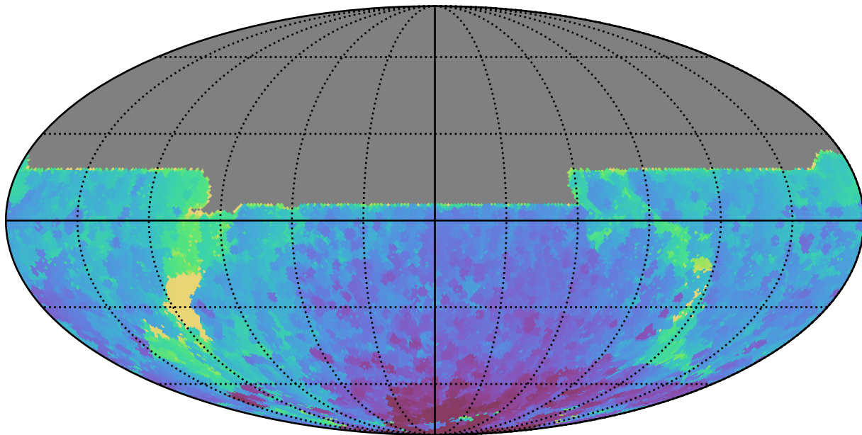
ddf_acor_sf10_lsf20_lsr50_v3.4_10yrs All sky y band: Min HA
