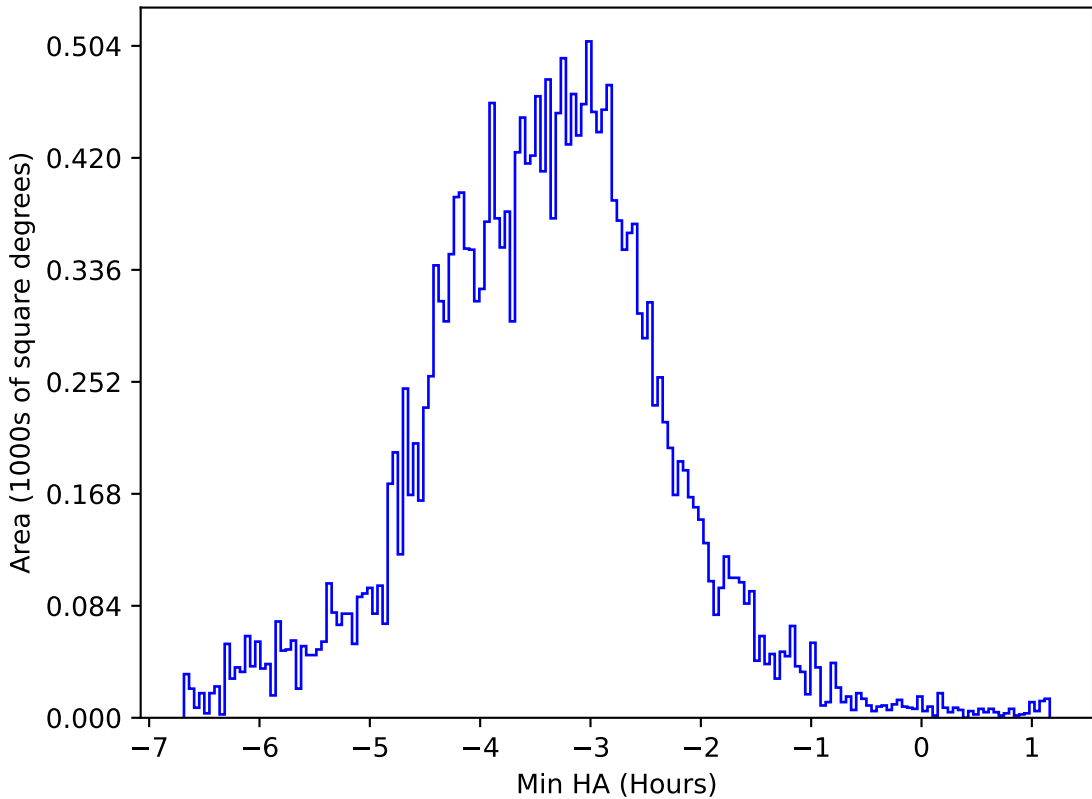
ddf_acor_sf10_lsf20_lsr50_v3.4_10yrs All sky y band: Min HA
