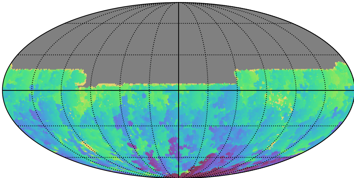
ddf_acor_sf10_lsf20_lsr50_v3.4_10yrs All sky u band: Min HA
