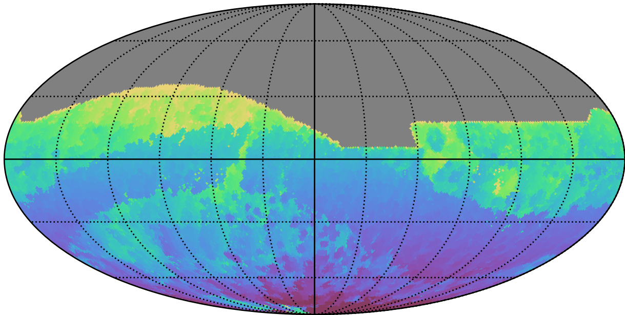
ddf_acor_sf10_lsf20_lsr50_v3.4_10yrs All sky r band: Min HA
