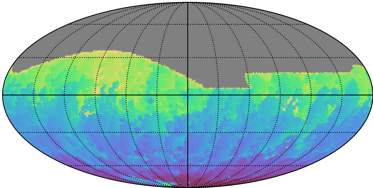
ddf_acor_sf10_lsf20_lsr50_v3.4_10yrs All sky g band: Min HA
