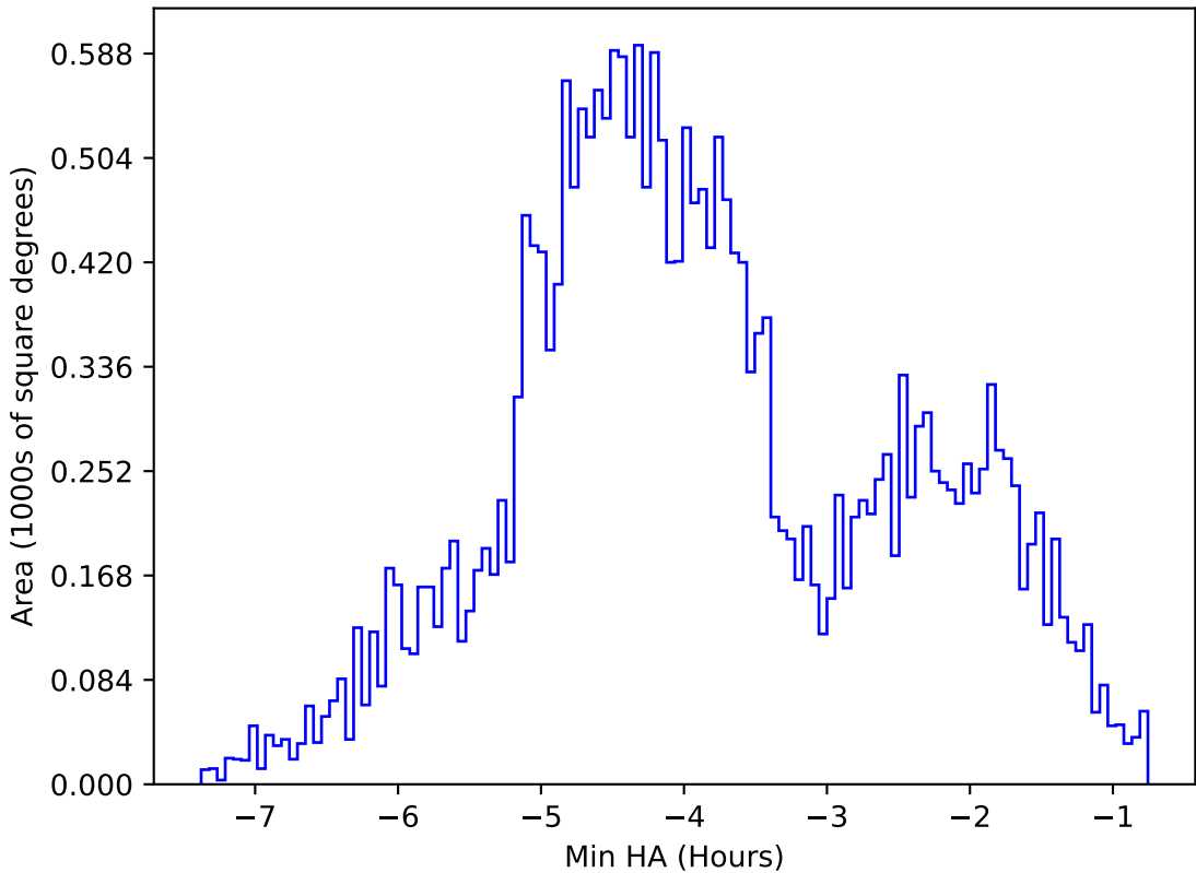
ddf_acor_sf10_lsf20_lsr50_v3.4_10yrs All sky g band: Min HA
