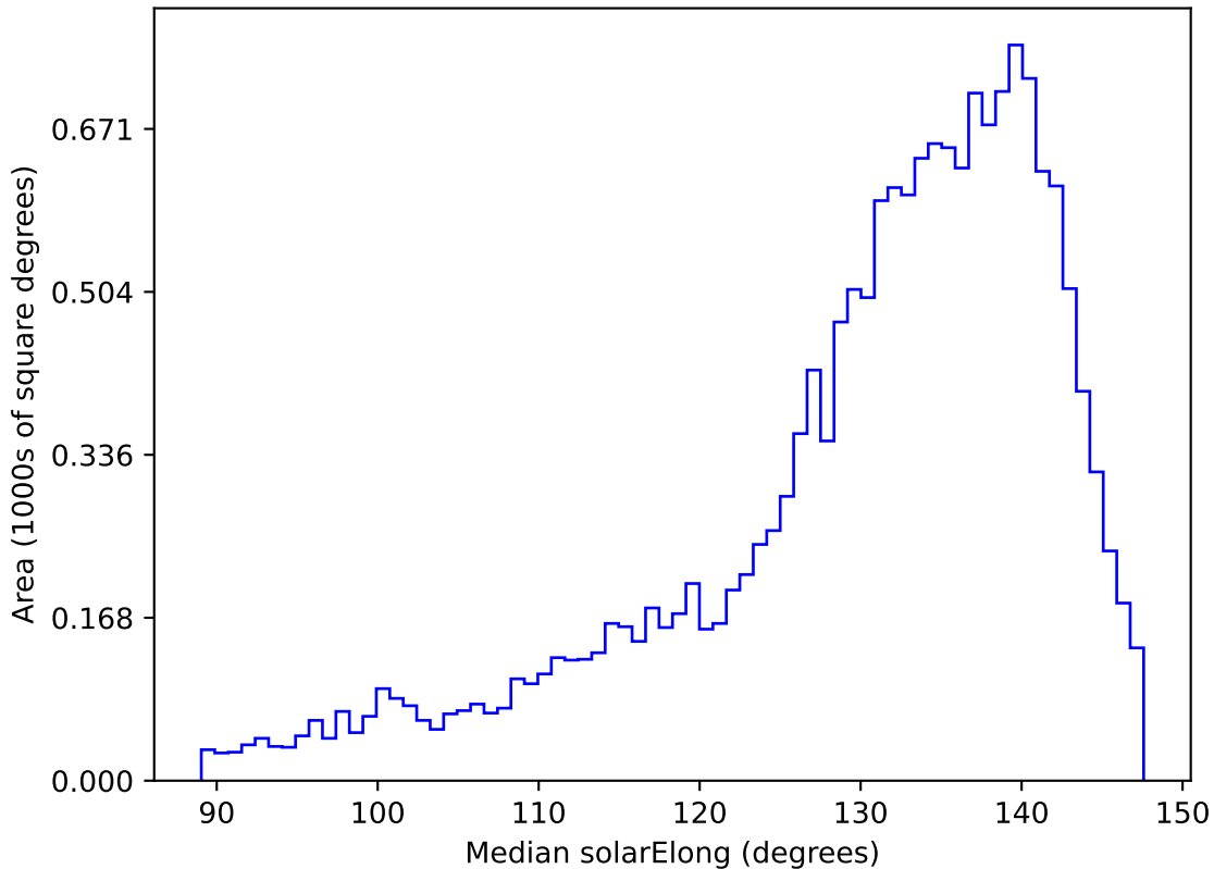
ddf_acor_sf10_lsf20_lsr50_v3.4_10yrs WFD y band: Median solarElong
