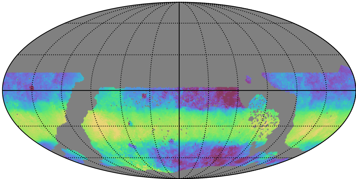
ddf_acor_sf10_lsf20_lsr50_v3.4_10yrs WFD y band: Median HA
