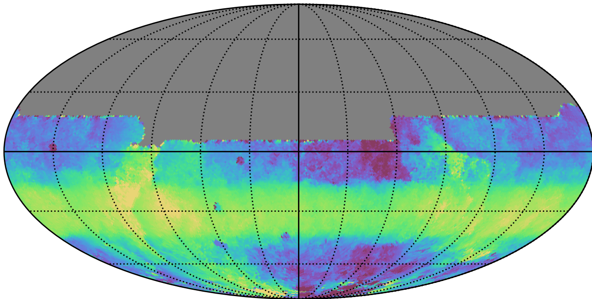
ddf_acor_sf10_lsf20_lsr50_v3.4_10yrs All sky y band: Median HA
