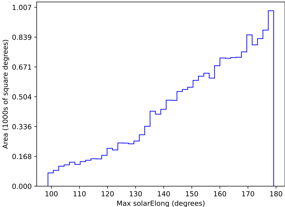
ddf_acor_sf10_lsf20_lsr50_v3.4_10yrs WFD y band: Max solarElong
