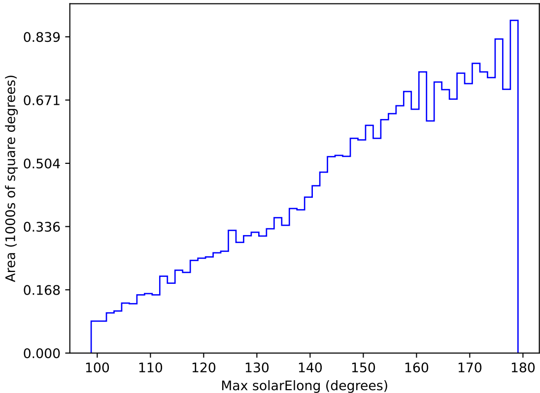
ddf_acor_sf10_lsf20_lsr50_v3.4_10yrs All sky y band: Max solarElong
