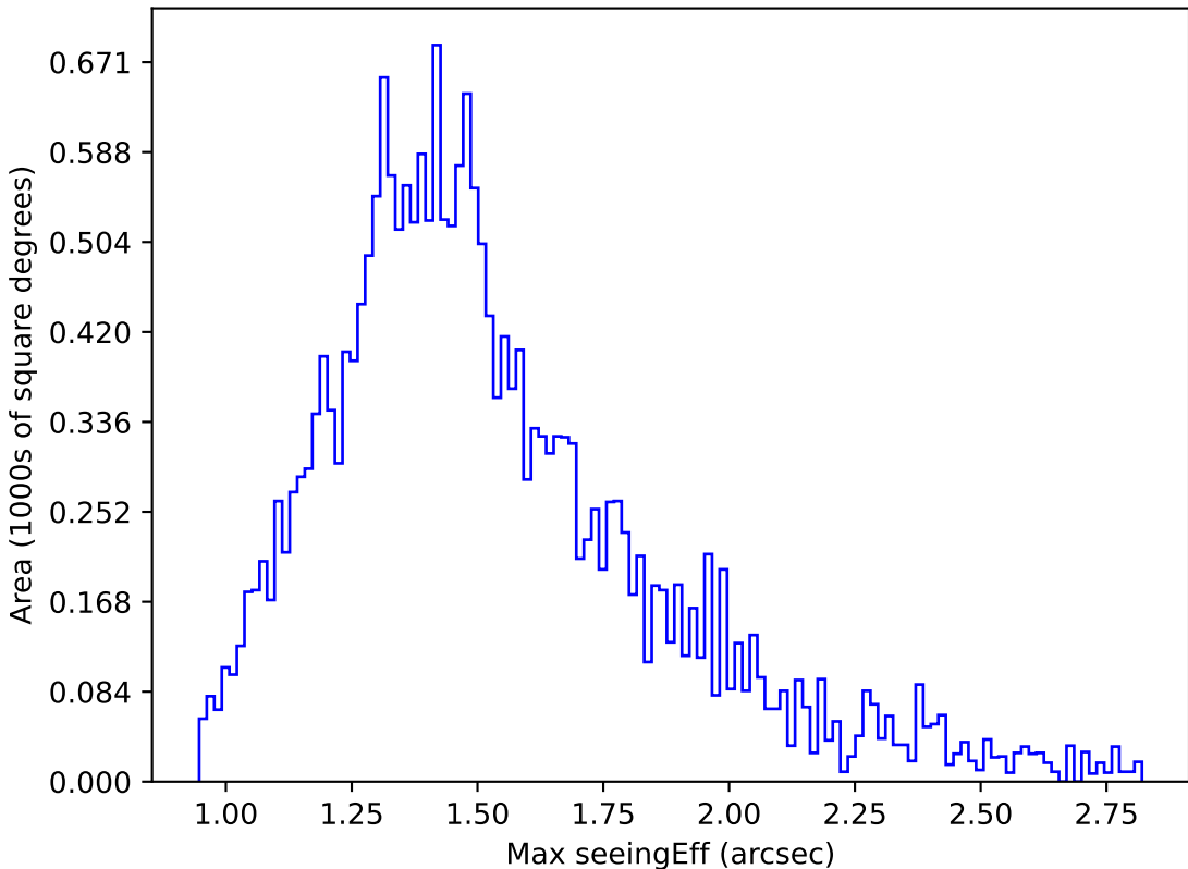
ddf_acor_sf10_lsf20_lsr50_v3.4_10yrs Yr 1 y band: Max seeingEff
