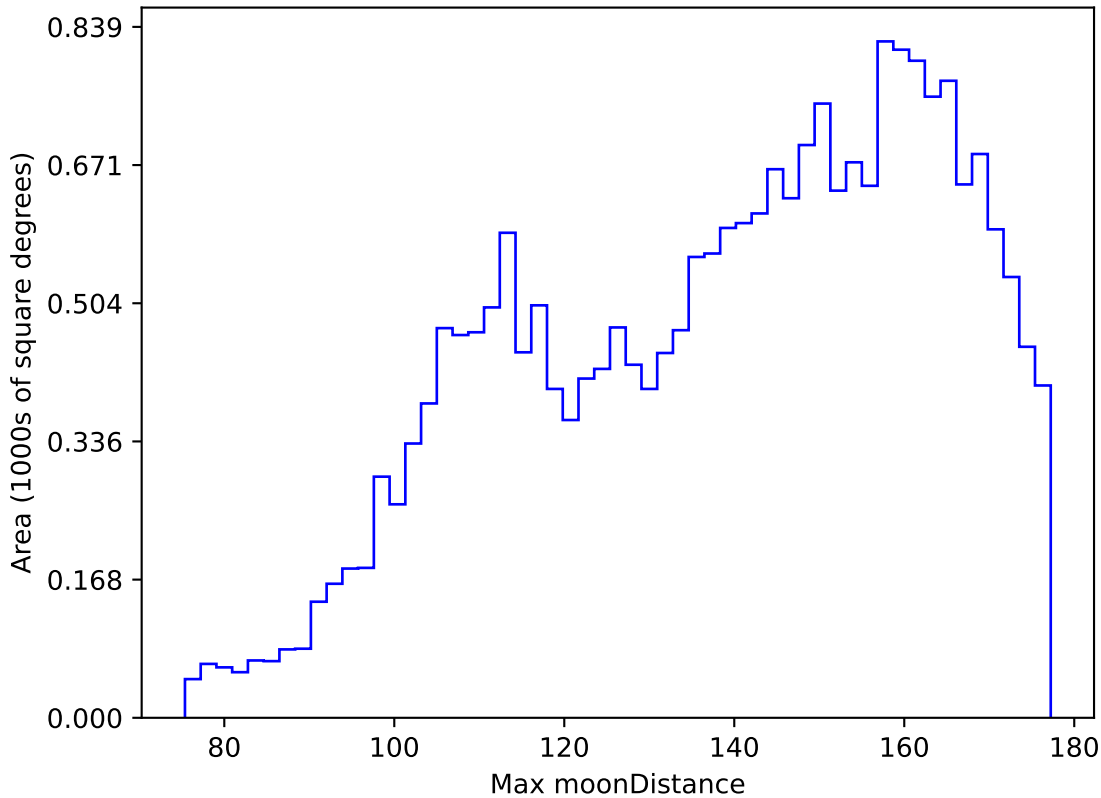
ddf_acor_sf10_lsf20_lsr50_v3.4_10yrs All sky y band: Max moonDistance
