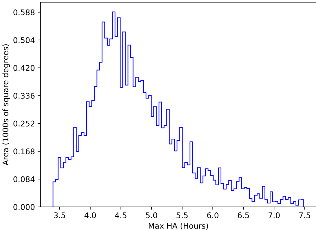
ddf_acor_sf10_lsf20_lsr50_v3.4_10yrs WFD y band: Max HA
