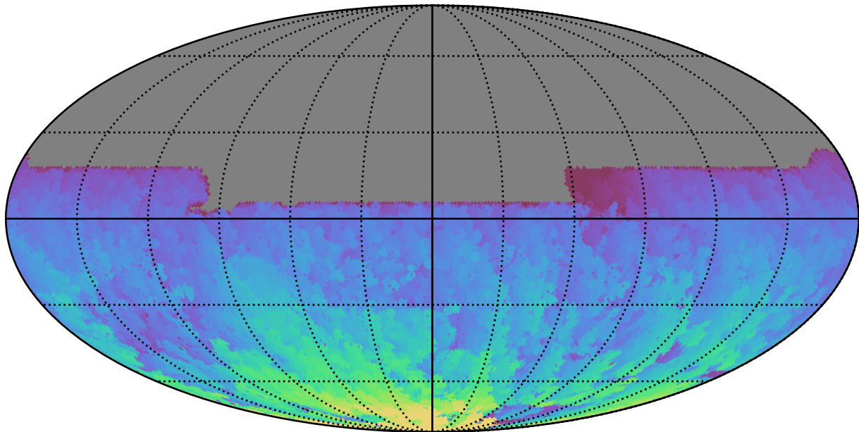
ddf_acor_sf10_lsf20_lsr50_v3.4_10yrs All sky y band: Max HA
