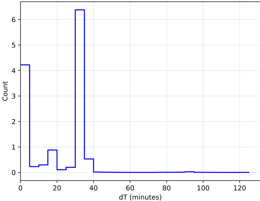
ddf_acor_sf10_lsf20_lsr50_v3.4_10yrs All sky: DeltaT Histogram
