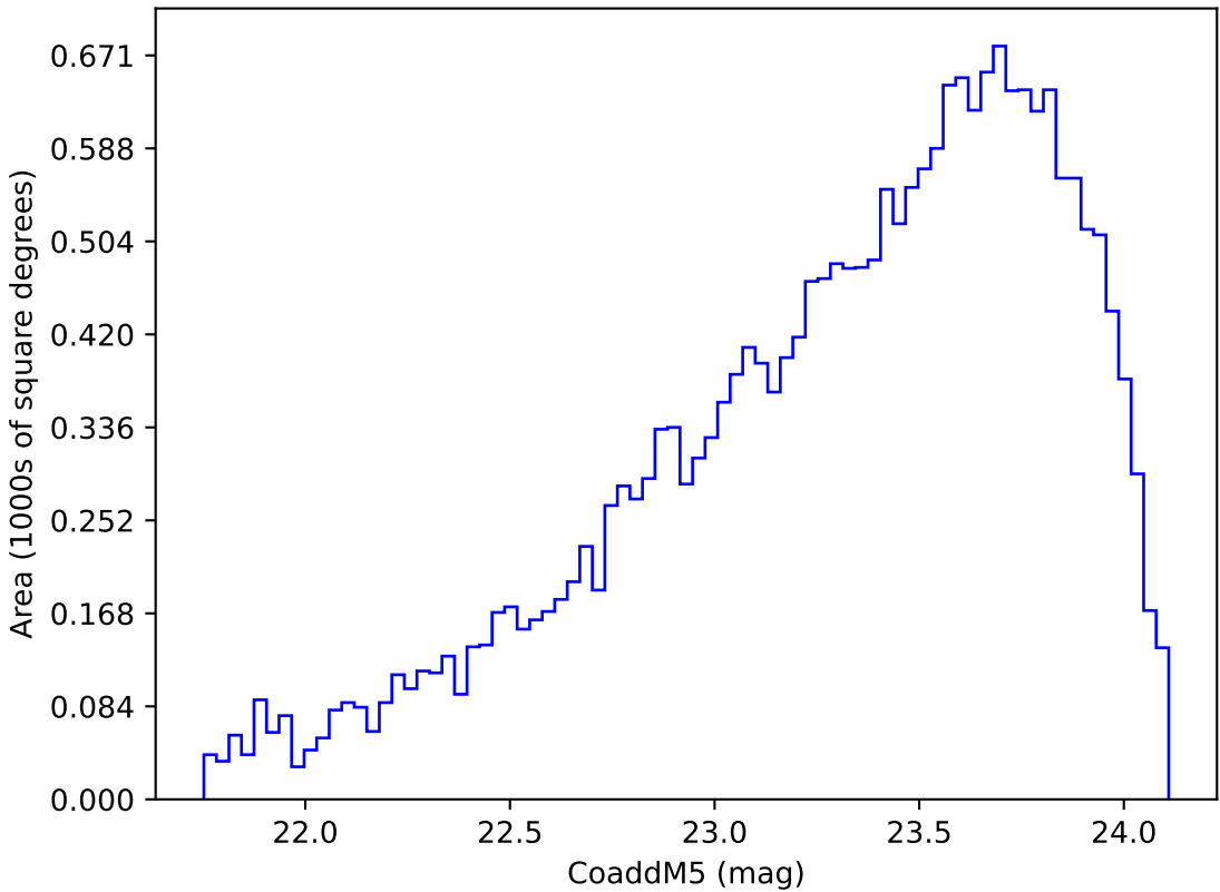
ddf_acor_sf10_lsf20_lsr50_v3.4_10yrs Yr 3-4 y band: CoaddM5
