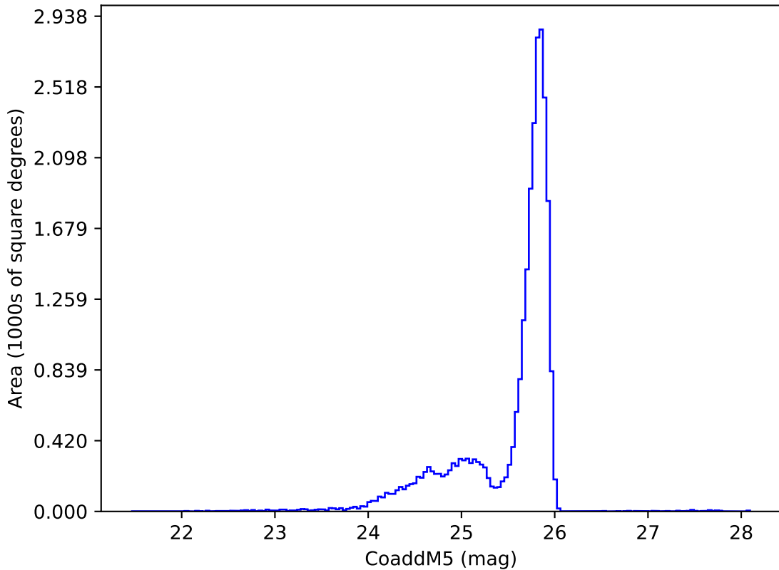
ddf_acor_sf10_lsf20_lsr50_v3.4_10yrs z: CoaddM5
