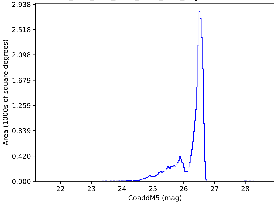
ddf_acor_sf10_lsf20_lsr50_v3.4_10yrs i: CoaddM5
