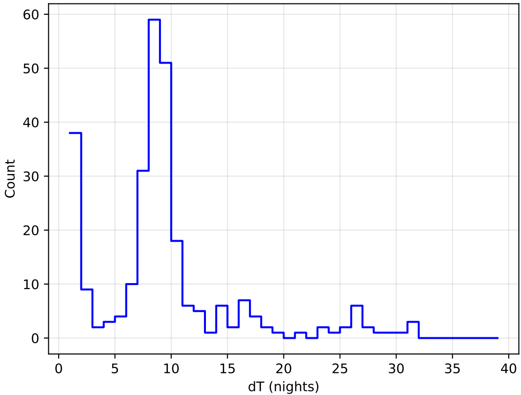
ddf_acor_sf10_lsf20_lsr50_v3.4_10yrs all bands: DD:ELAISS1 Delta Nights Histogram
