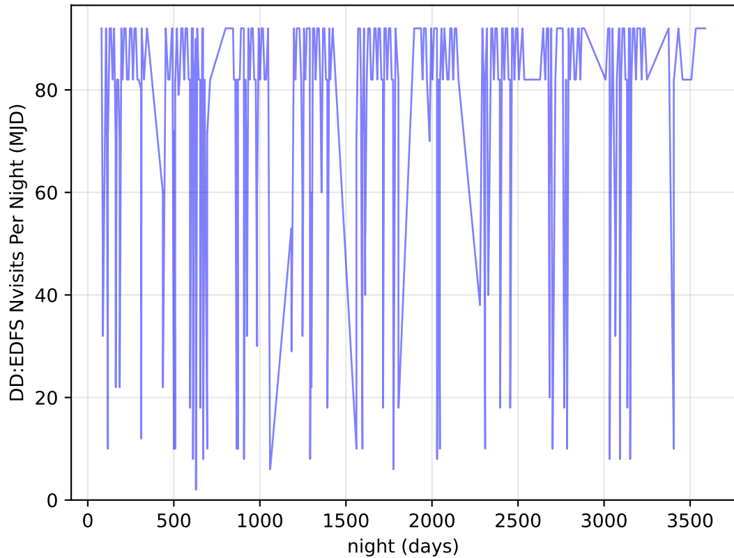
ddf_acor_sf10_lsf20_lsr50_v3.4_10yrs all bands: DD:EDFS Nvisits Per Night
