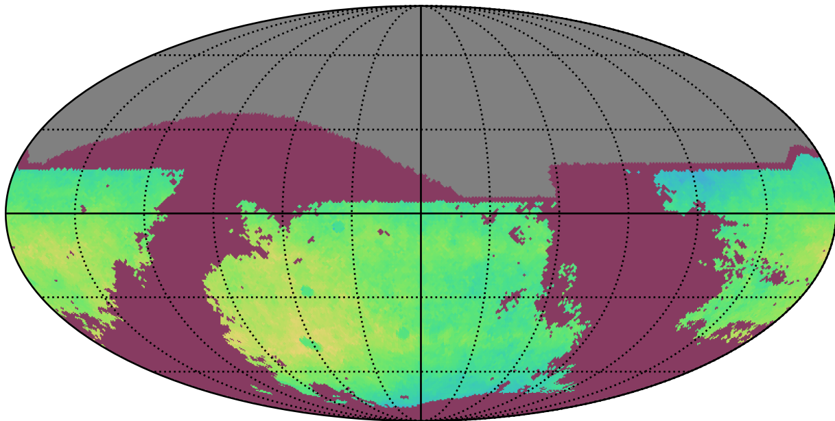
ddf_acor_sf10_lsf20_lsr20_v3.4_10yrs i: NgalScale
