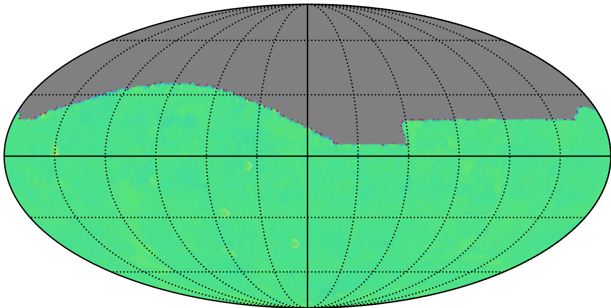
ddf_acor_sf10_lsf20_lsr20_v3.4_10yrs i: Kuiper rotTelPos
