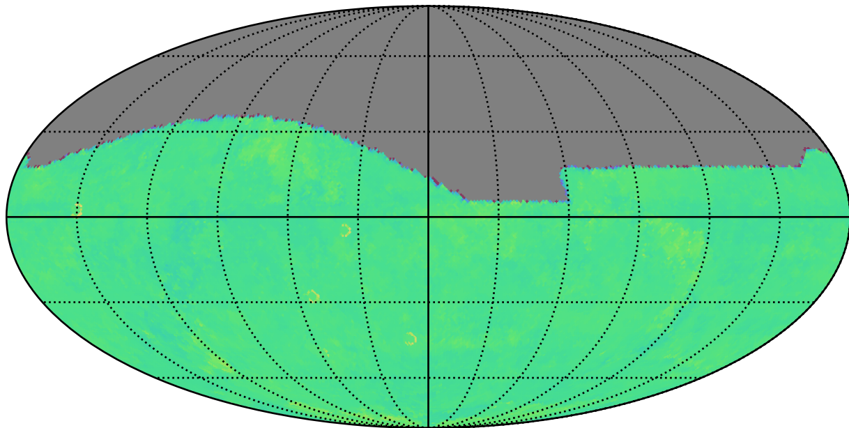
ddf_acor_sf10_lsf20_lsr20_v3.4_10yrs g: Kuiper rotTelPos
