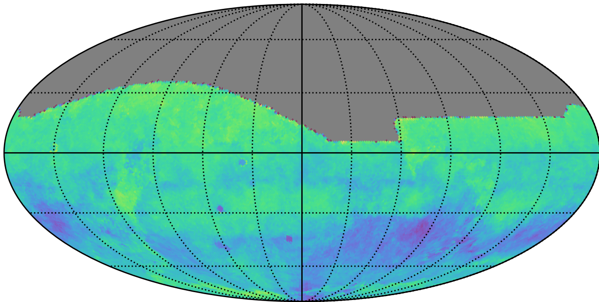
ddf_acor_sf10_lsf20_lsr20_v3.4_10yrs i: Kuiper rotSkyPos
