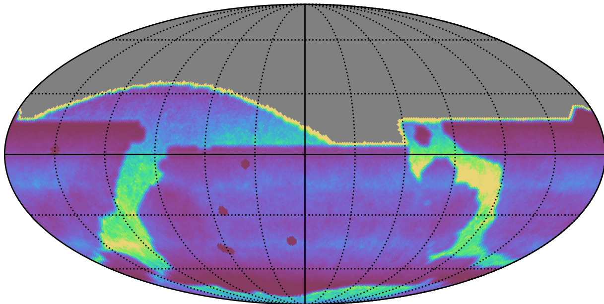
ddf_acor_sf10_lsf20_lsr20_v3.4_10yrs : DCRprecision
