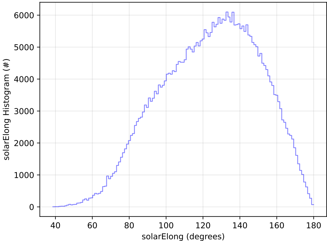
ddf_acor_sf10_lsf20_lsr20_v3.4_10yrs All sky y band: solarElong Histogram
