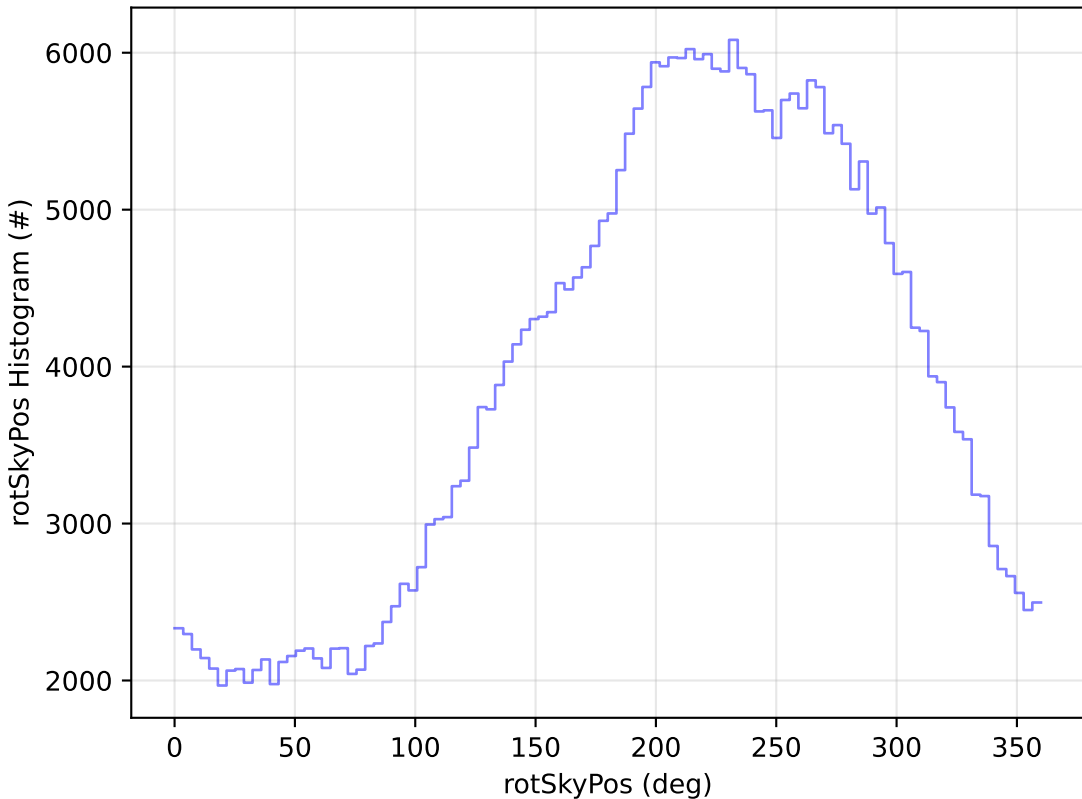
ddf_acor_sf10_lsf20_lsr20_v3.4_10yrs All sky y band: rotSkyPos Histogram
