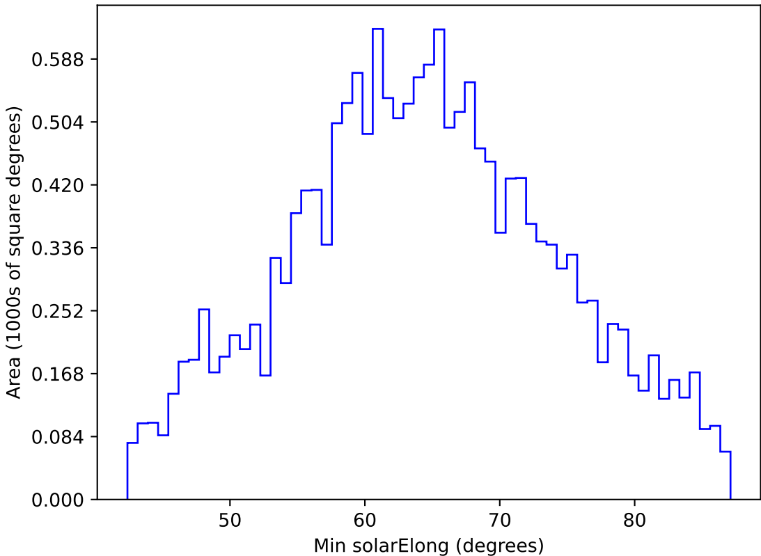
ddf_acor_sf10_lsf20_lsr20_v3.4_10yrs WFD y band: Min solarElong
