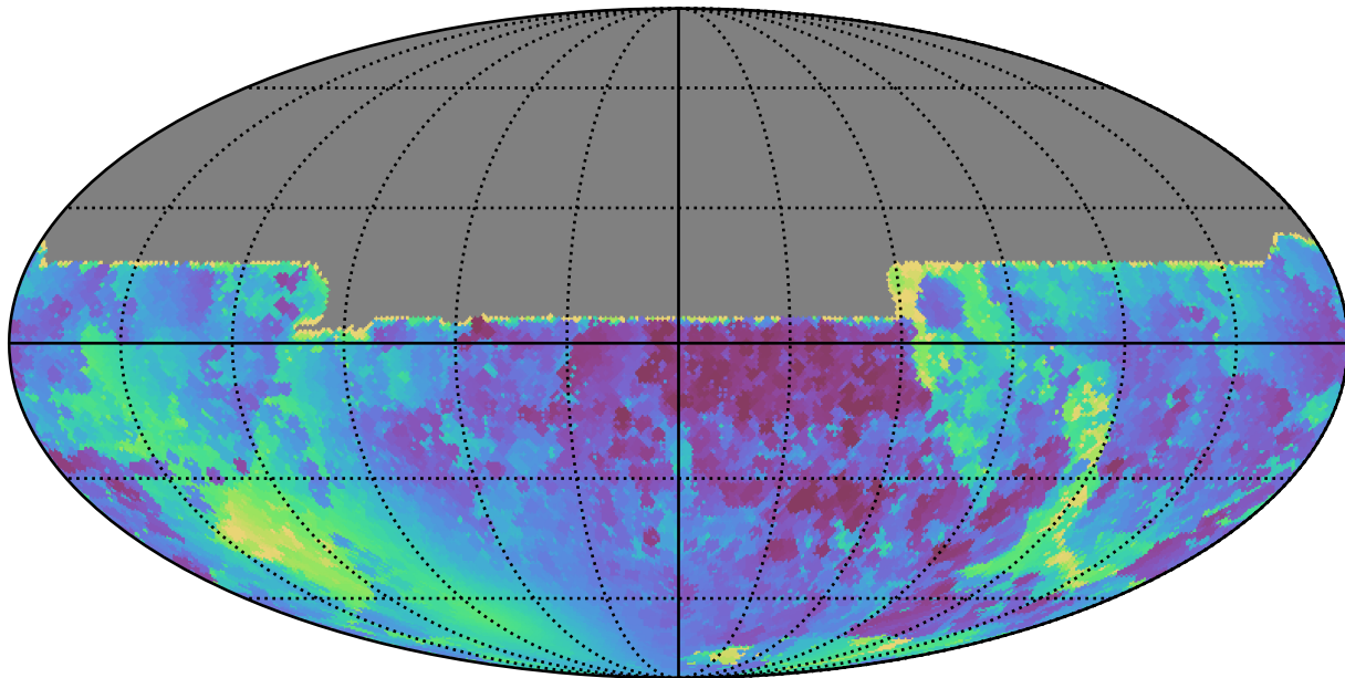
ddf_acor_sf10_lsf20_lsr20_v3.4_10yrs All sky y band: Min solarElong
