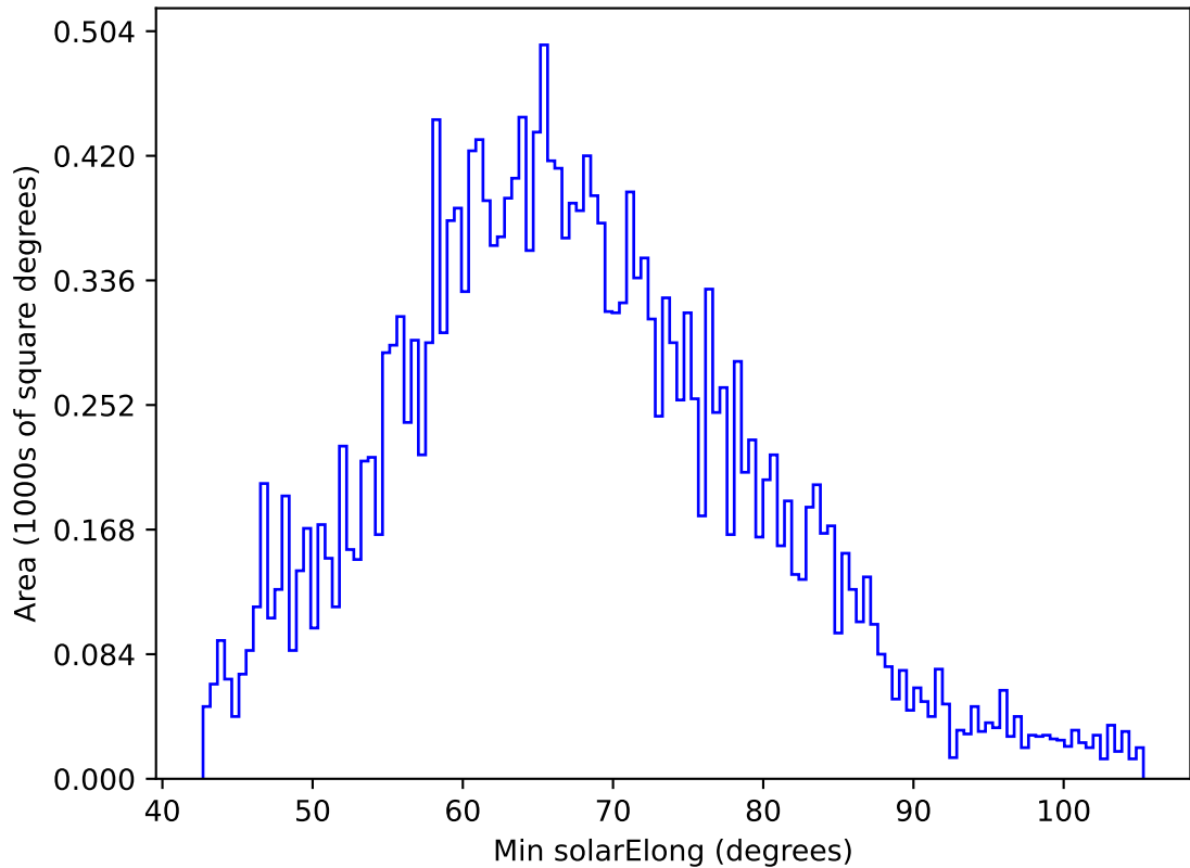
ddf_acor_sf10_lsf20_lsr20_v3.4_10yrs All sky y band: Min solarElong
