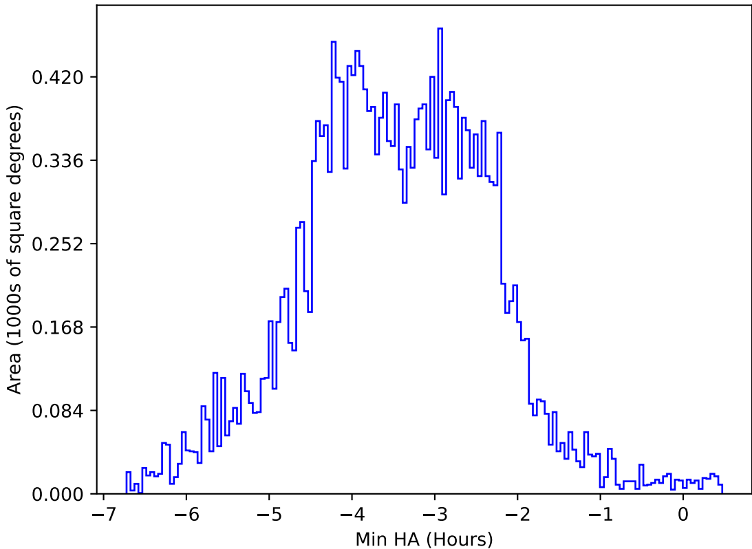
ddf_acor_sf10_ls20_lsr20_v3.4_10yrs All sky y band: Min HA
