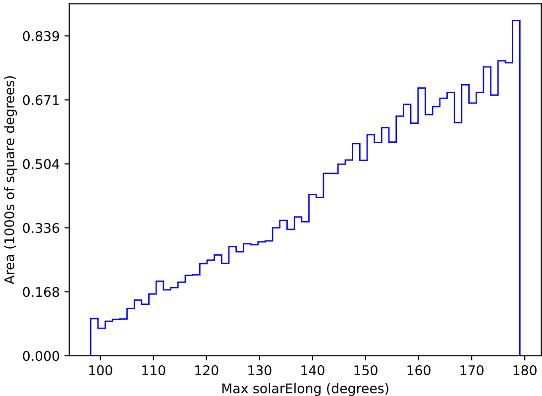
ddf_acor_sf10_lsf20_lsr20_v3.4_10yrs All sky y band: Max solarElong
