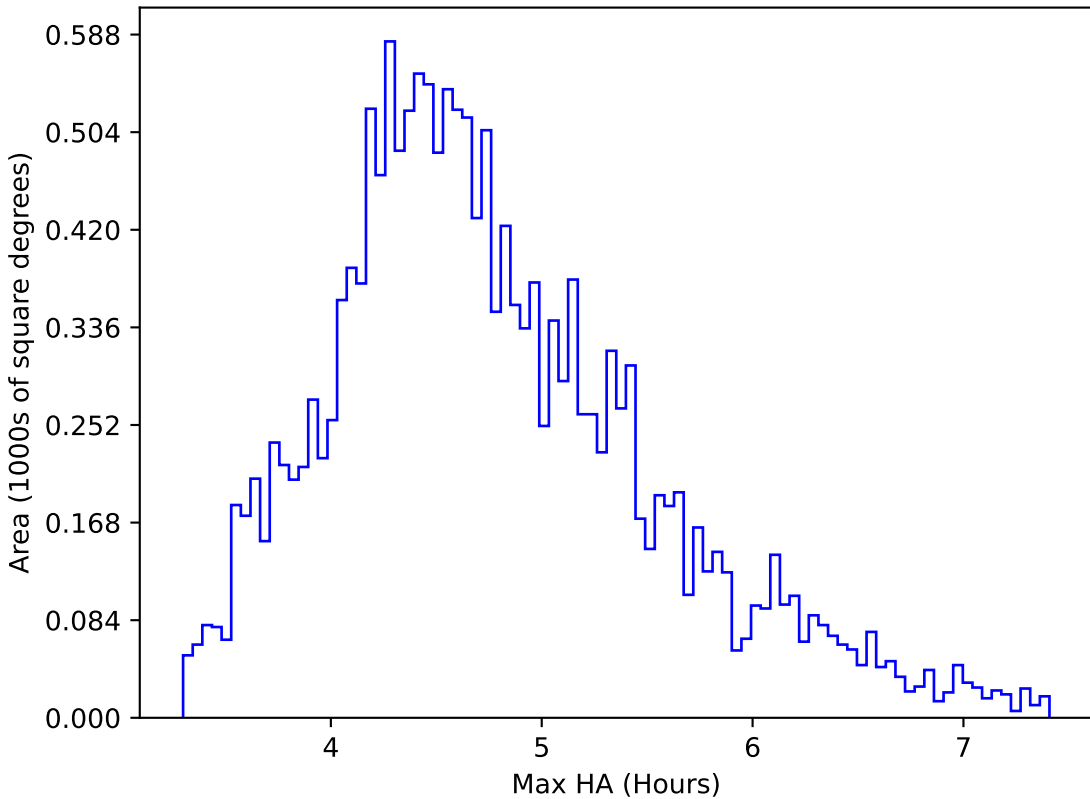
ddf_acor_sf10_lsf20_lsr20_v3.4_10yrs WFD y band: Max HA
