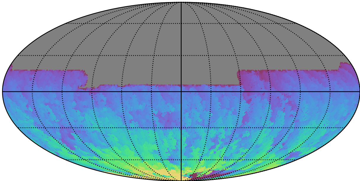
ddf_acor_sf10_lsf20_lsr20_v3.4_10yrs All sky y band: Max HA
