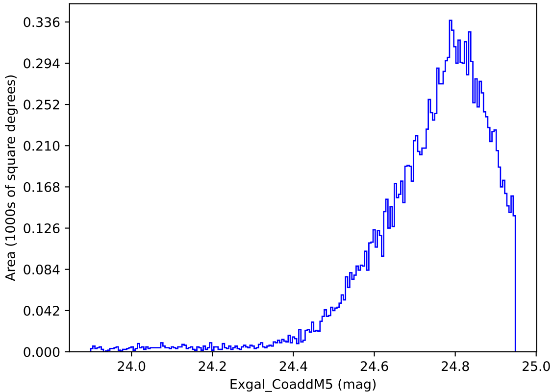
ddf_acor_sf10_lsf20_lsr20_v3.4_10yrs WFD y band: Exgal_CoaddM5
