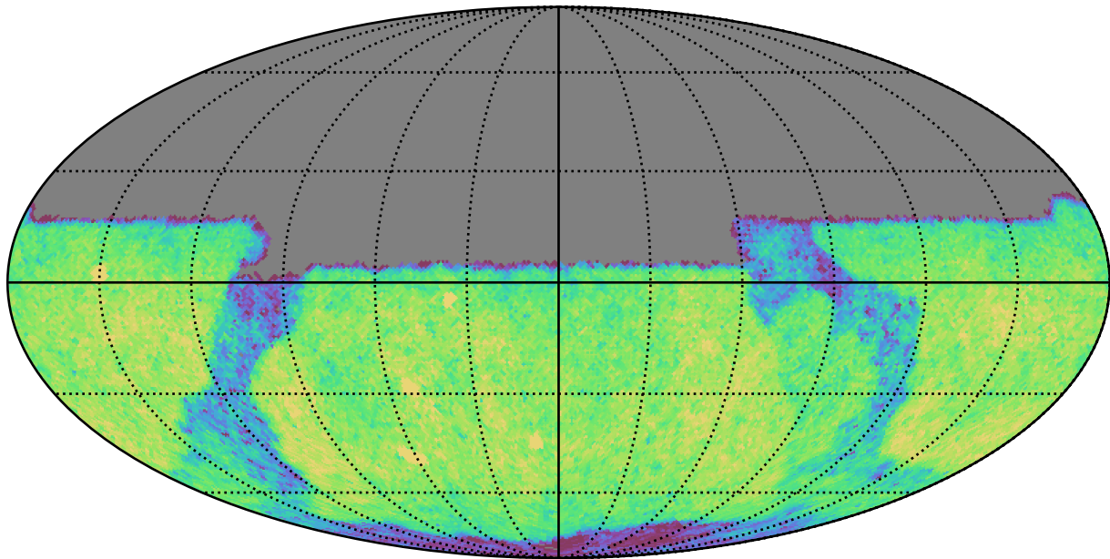
ddf_acor_sf10_lsf20_lsr20_v3.4_10yrs Yr 1 y band: CoaddM5
