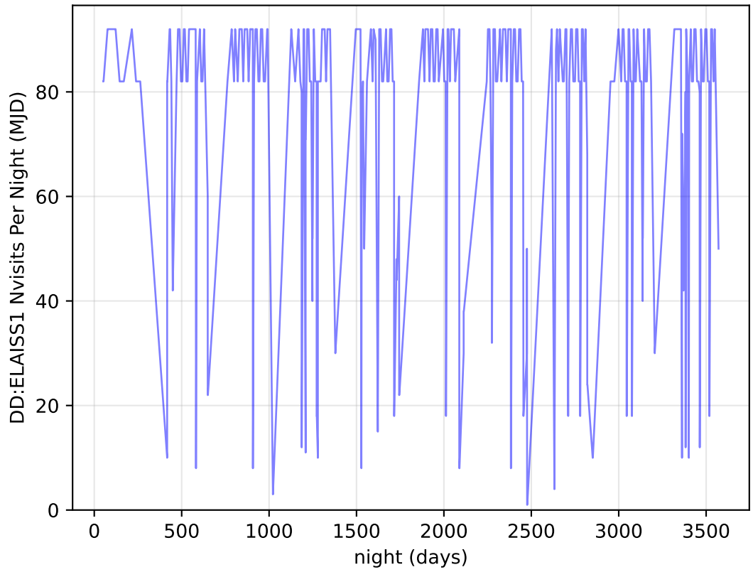
ddf_acor_sf10_ls10_lsr20_v3.4_10yrs all bands: DD:ELAISS1 Nvisits Per Night
