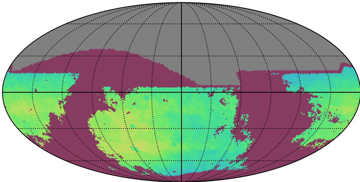
ddf_acor_sf10_lsf20_lsr10_v3.4_10yrs i: NgalScale
