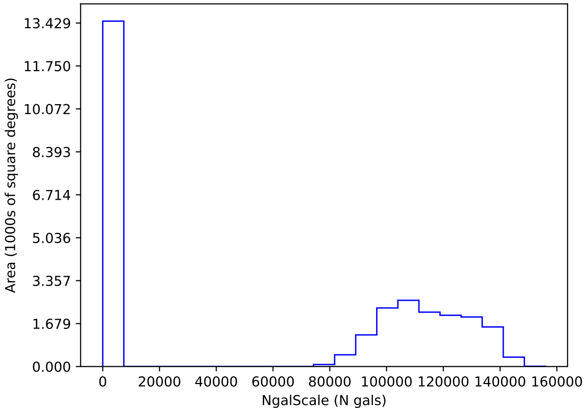
ddf_acor_sf10_lsf20_lsr10_v3.4_10yrs i: NgalScale
