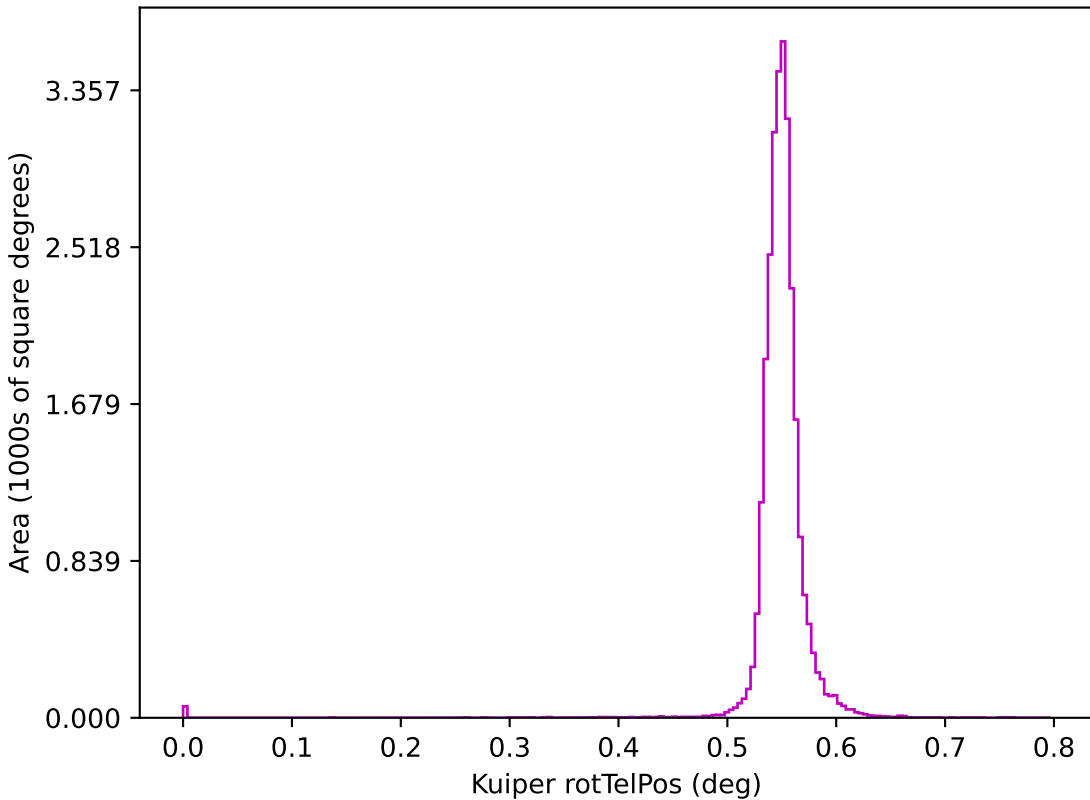
ddf_acor_sf10_lsf20_lsr10_v3.4_10yrs z: Kuiper rotTelPos
