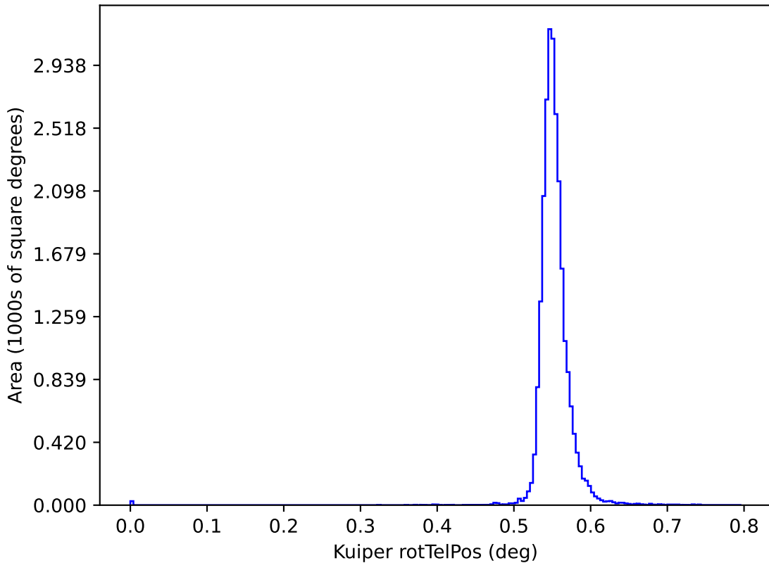
ddf_acor_sf10_lsf20_lsr10_v3.4_10yrs y: Kuiper rotTelPos
